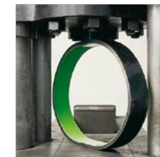
Gracias a su elasticidad, el poliuretano se mantiene intacto frente a una deformación de la tubería.
